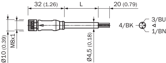
尺寸图 (尺寸单位: mm)
