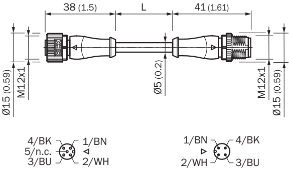
尺寸图 (尺寸单位: mm)
