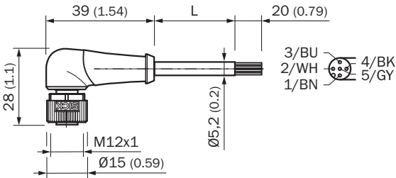
尺寸图 (尺寸单位: mm)
