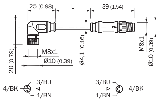
尺寸图 (尺寸单位: mm)
