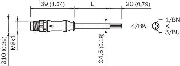
尺寸图 (尺寸单位: mm)
