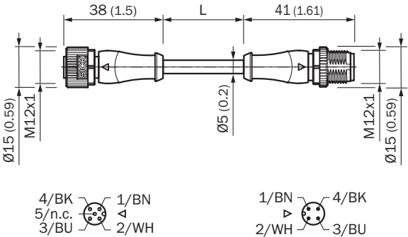
尺寸图 (尺寸单位: mm)
